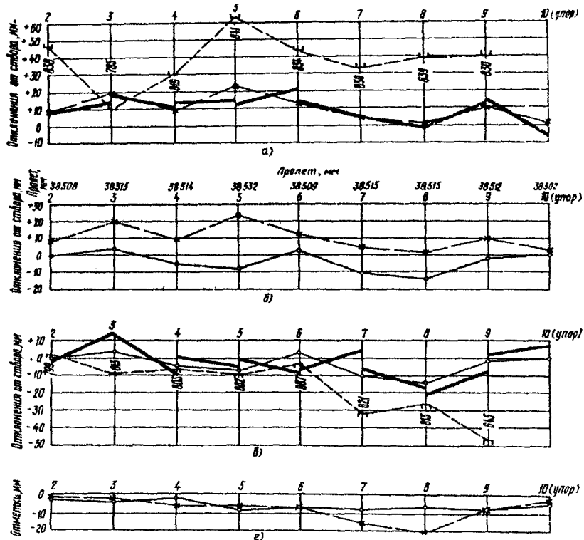
а - положение рельсов, балок и граней колонн ряда Б; б - совместное плановое положение осей рельсов А и Б; в - положение рельсов, балок и граней колонн ряда А; г - профиль подкранового пути
