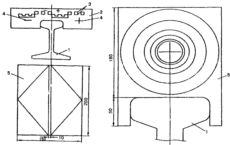
1 - рельс; 2 - шаблон со шкалой; 3 - деления шкалы 10×10 мм; 4 - знак шкалы; 5 - визирная марка
