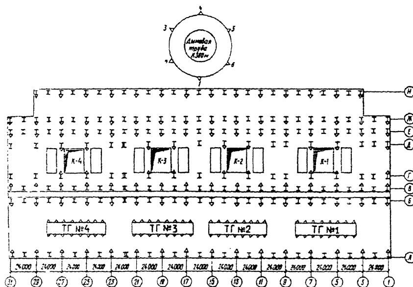
Рисунок 5 - Схема размещения марок в главном корпусе ГРЭС с энергоблоками 800 МВт
